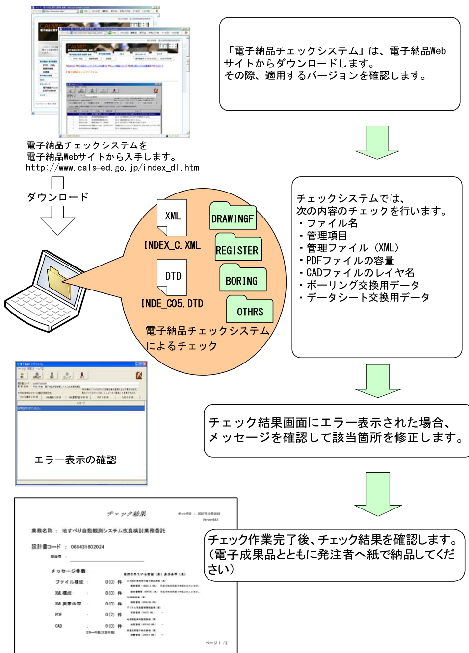
図 5-14 電子納品チェックシステムを用いた電子成果品のチェック
